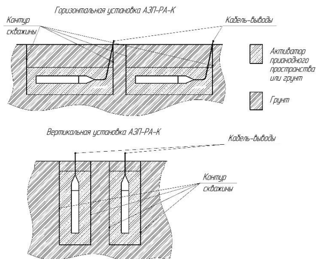
Установка АЗП-РА-К
