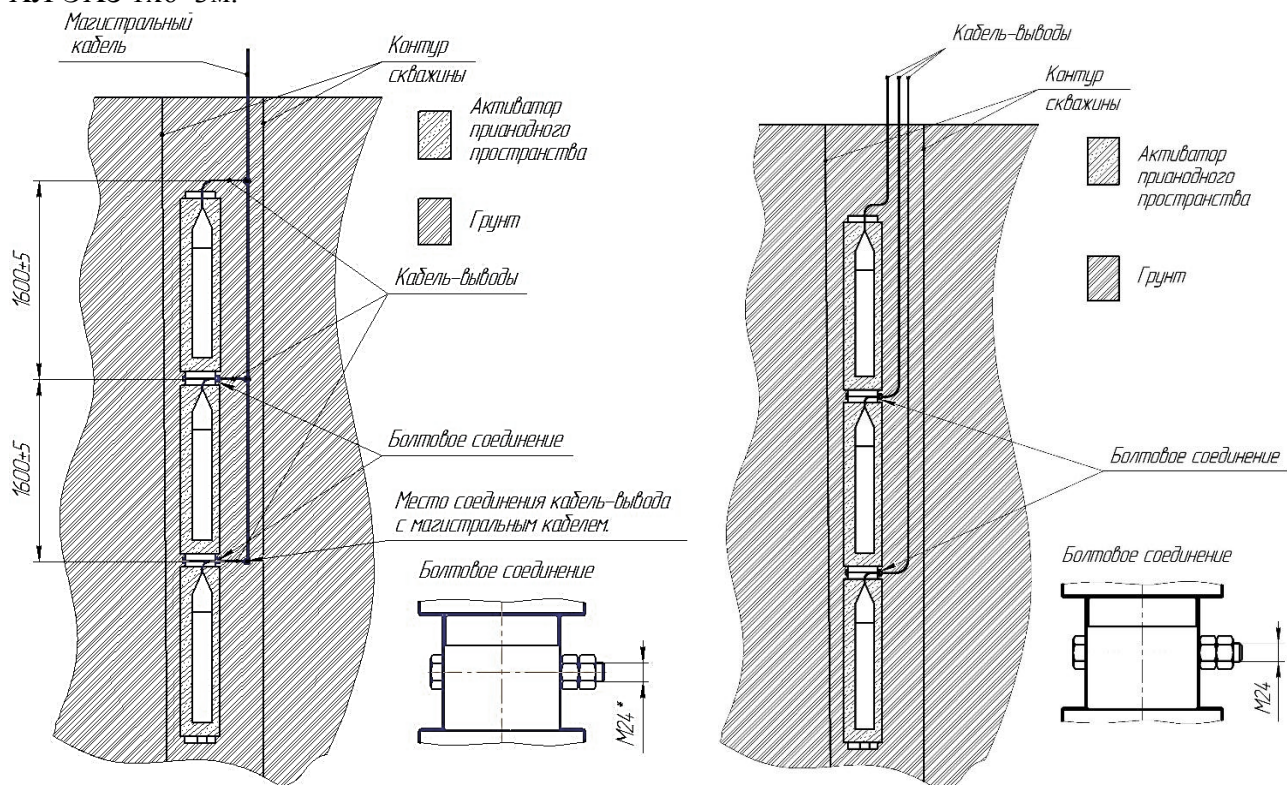
Установка АЗП-РА-ГУ в скважину с магистральным кабелем
