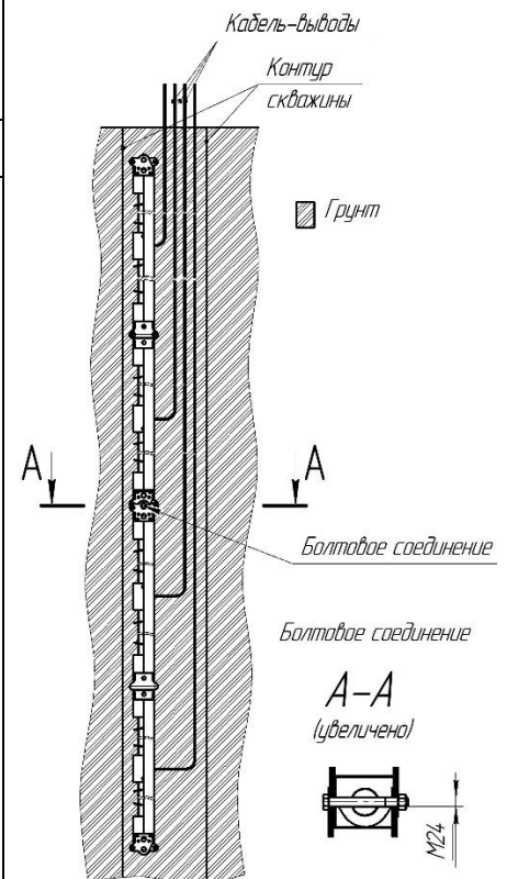
Установка АЗП-РА-ГС в грунт без магистрального кабеля
